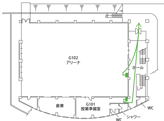
1階平面図
